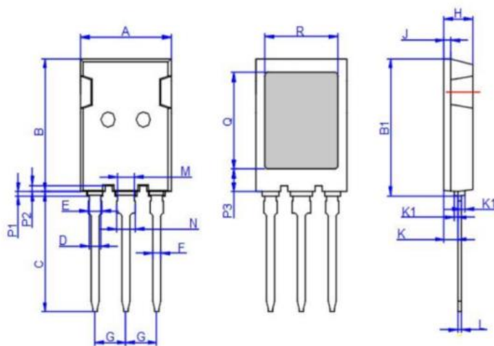
TO-247iPS-3L
